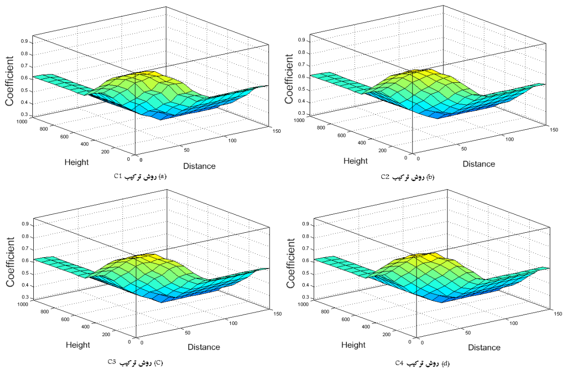
شکل ۱۱- سطح بوجود آمده بین توابع عضویت فازی فاصله و ارتفاع
