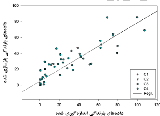
شکل ۸- مقایسه داده‌های بارندگی بازسازی شده و مشاهده‌ای در ایستگاه تربت‌حیدریه
