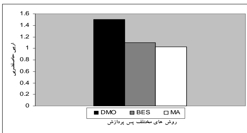
شکل ۵- اربیی حاصلضربی برون داد خام مدل و برون داد پس پردازش شده
