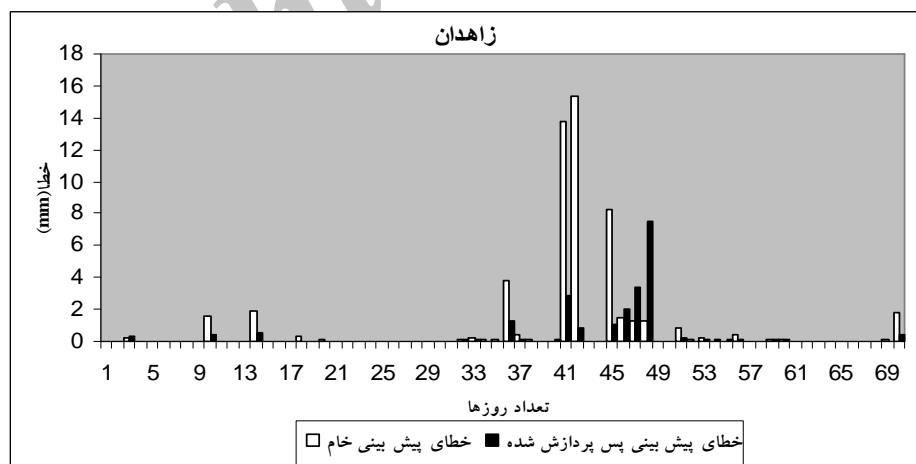
شکل ۳- خطای مطلق پیش‌بینی خام و پس‌پردازش شده مدل برای روزهای مختلف، برای ایستگاه‌های هم‌دید اردبیل، یاسوج و زاهدان
