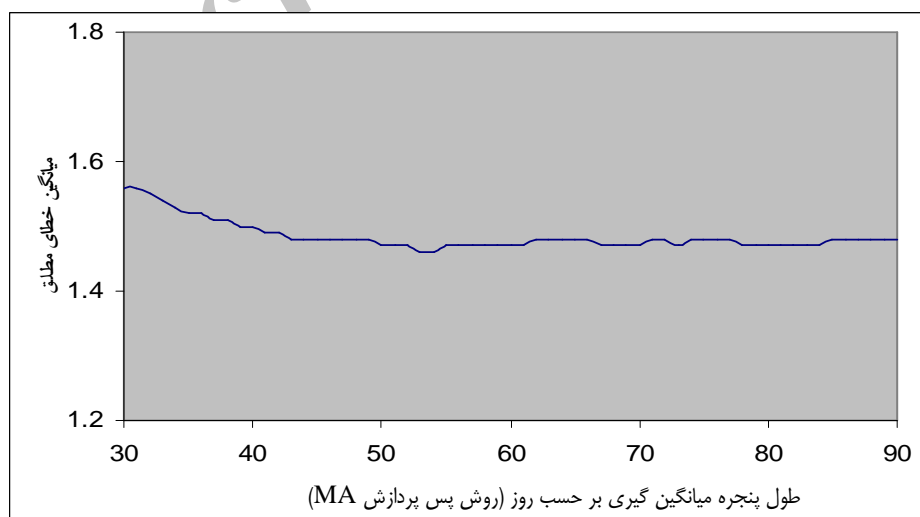
شکل ۲- میانگین خطای مطلق پیش‌بینی بارندگی‌های ۲۴ ساعته (برحسب میلی‌متر)، به عنوان تابعی از طول پنجره میانگین گیری
