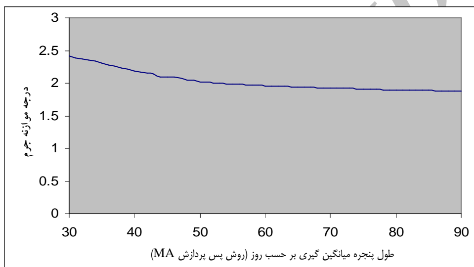
شکل ۱- میانگین درجه موازنه جرم برای بارش‌های ۲۴ ساعته برای ۲۰۵ ایستگاه همدید کشور
