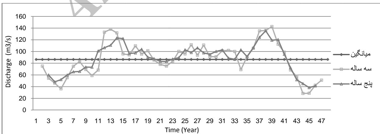
شکل ۴- میانگین آبدهی سالانه و میانگین متحرک ۳ و ۵ ساله ورودی سد شهریار
