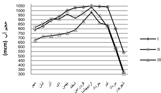
شکل ۶- مقایسه حجم آب (mcm) در مخزن سد سفیدرود، مدل‌های I, II, III
