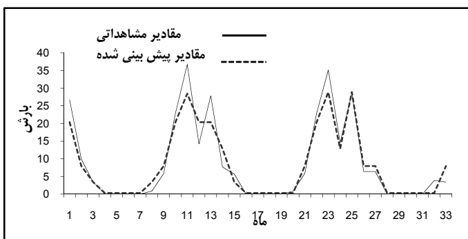
شکل ۹- نمودار تغییرات مقادیر پیش‌بینی شده در مقابل مقادیر واقعی با استفاده از داده‌های میانگین متحرک پنج ساله داده‌ها
