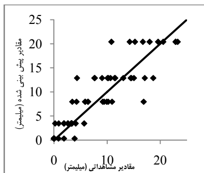
شکل ۹- نمودار تغییرات مقادیر پیش‌بینی شده در مقابل مقادیر واقعی با استفاده از داده‌های میانگین متحرک پنج ساله داده‌ها
