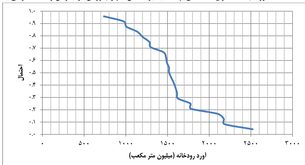
شکل ۵- توزیع تجمعی احتمال آورد سالیانه سد زاینده رود
