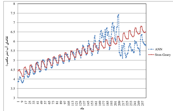
شکل ۵- مقایسه تقاضای سرانه آب پیش‌بینی شده با مدل استون‌گیری و شبکه عصبی برای دوره‌ی ۱۳۹۰-۱۴۱۰
