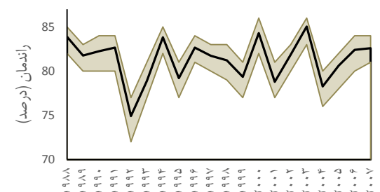
شکل ۶- باند عدم قطعیت راندمان حوضه‌ای (وضع موجود آبیاری)
