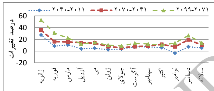
شکل ۳- درصد تغییرات دمای ماهانه و سالانه زیر حوضه مطالعاتی تحت دو سناریو: الف) A2 و ب) B1
