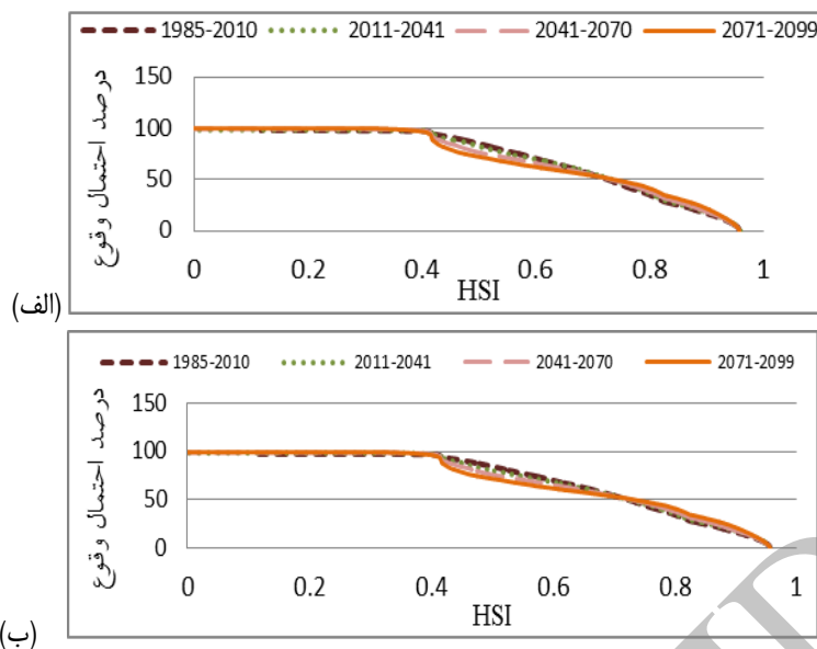
شکل ۱۲- مقایسه احتمال وقوع HSI های مختلف طی ۱۰۰ سال آتی با دوره پایه تحت دو سناریو: الف) A2 و ب) B1
