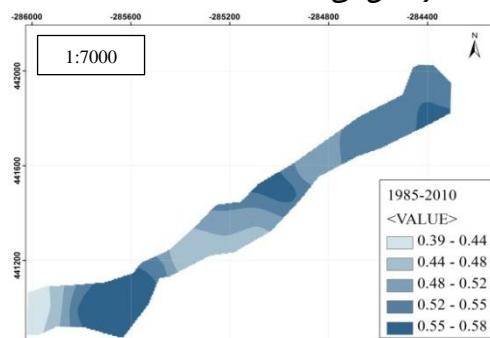
شکل ۹- مطلوبیت زیستگاه (HSI) سگ ماهی جوپاری در دوره ۲۰۱۰-۱۹۸۵
