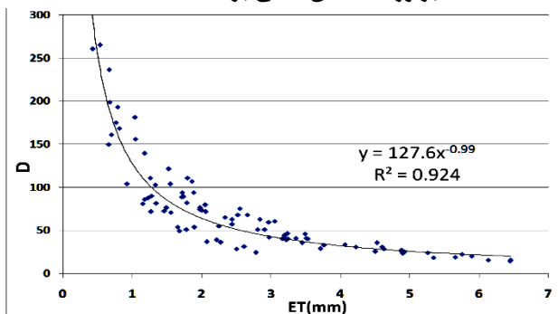
شکل ۳- حساسیت تبخیر (ET) به ۵۰ درصد افزایش در برآورد آلبیدو سطحی-α
