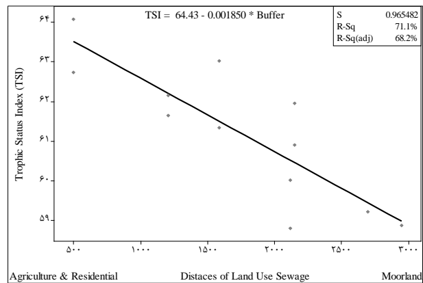
شکل ۶- رگرسیون مدل تغذیه‌گرایی سطح تالاب چغاور با پساب‌های کاربری اراضی، سالهای ۸۳-۸۵
