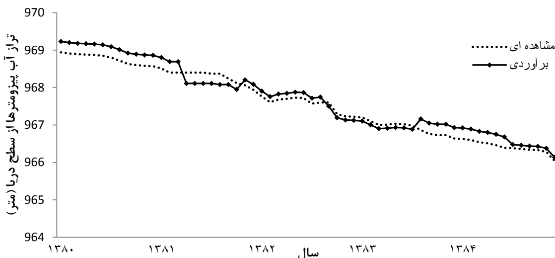
شکل ۶- نتایج صحت‌سنجی مدل ناپایدار آبخوان یزد- اردکان
