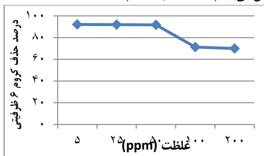
شکل ۴ - اثر غلظت اولیه کروم بر روی کارایی حذف کروم ۶ ظرفیتی (pH=۳، مقدار ماده جاذب ۳ گرم، زمان تماس ۱۲۰ دقیقه و دما ۲۲ درجه سانتی گراد)
