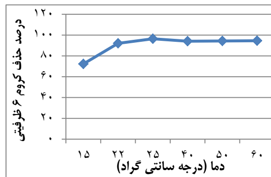
شکل ۵- اثر دما بر روی کارایی حذف (pH=۳)، مقدار ماده جاذب ۳ گرم، غلظت اولیه کروم ۵ mg/l و زمان تماس ۱۲۰ دقیقه
