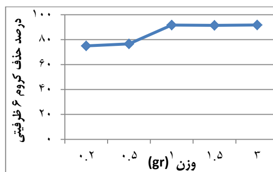
شکل ۳- اثر وزن جاذب در راندمان حذف کروم شش ظرفیتی (pH=۳، غلظت اولیه کروم ۵۰ mg/l، زمان تماس ۱۲۰ دقیقه و دما ۲۲ درجه سانتی گراد)
