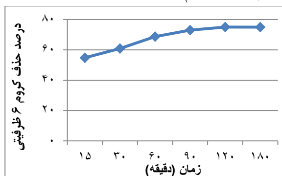
شکل ۲- تأثیر زمان تماس بر روی کارایی حذف کروم ۶ ظرفیتی (pH=۳، مقدار ماده جاذب ۰/۲ گرم، غلظت اولیه کروم شش ظرفیتی ۵۰ mg/l و دما ۲۲ درجه سانتی گراد)
