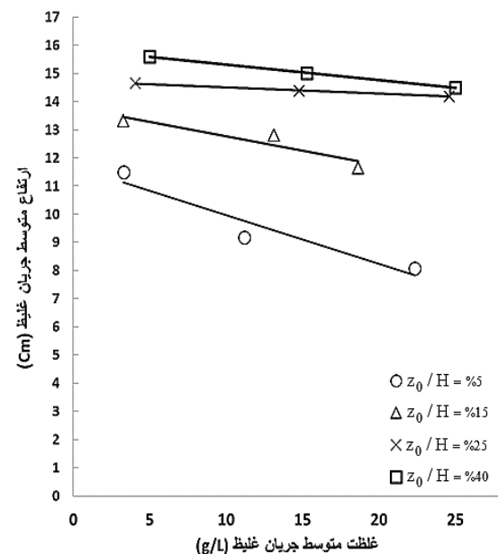
شکل ۹- نمودار تغییرات ضخامت جریان غلیظ در مقابل غلظت جریان غلیظ در وضعیت‌های مختلف دریاچه تخلیه
