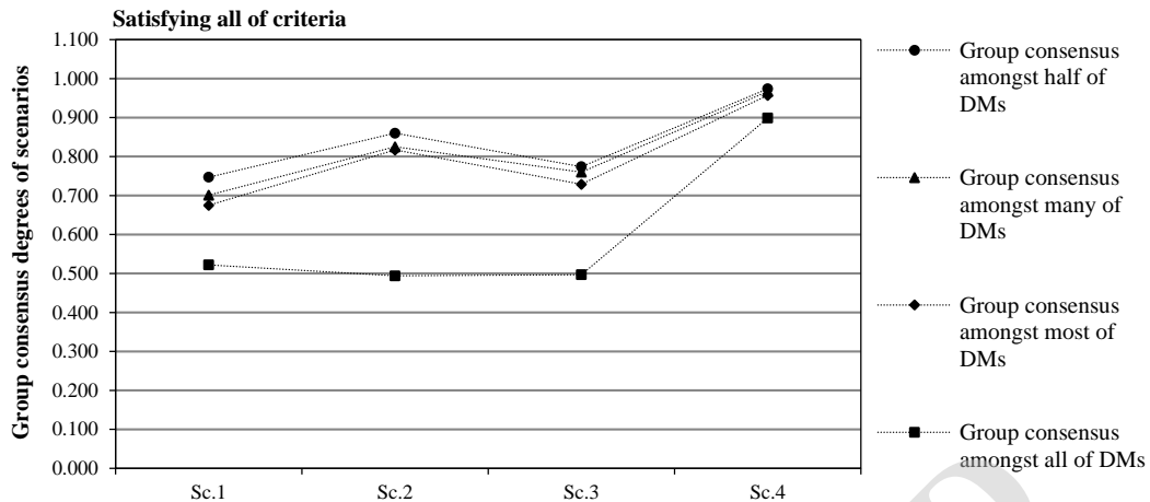
Fig. 7. Group consensus degrees of scenarios in the second type several risk cases شکل ۷- درجه اجماع گروهی طرح‌ها در حالت‌های مختلف ریسک نوع دوم
