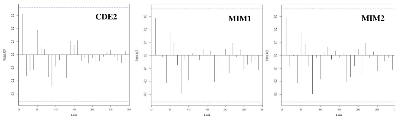
Fig. 4. ACF and PACf for CDE2, MIM1 and MIM2 models for exploring the number of p in AR (p) model شکل ۴- نمودار PACF برای شناسایی عدد p در مدل AR(p) برای مدل های CDE2، MIM1 و MIM2
