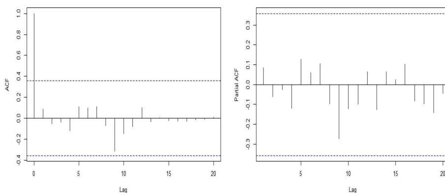
Fig3: ACF and PACf plots after calculating of correlation شکل ۳- نمودار ACF و PACF بعد از اجرای مدل سری زمانی در مدل CDE1
