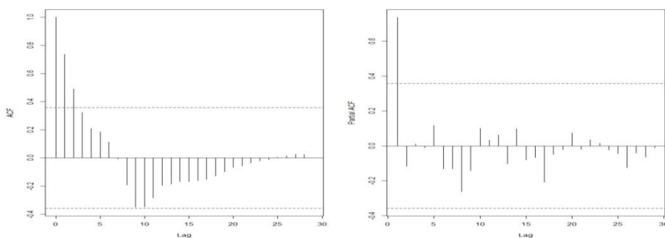
Fig. 2. ACF and PACf plots for exploring the number of p in AR (p) model(CDE1) شکل ۲- نمودار ACF و PACF برای شناسایی عدد p در مدل AR(p) برای مدل CDE1
