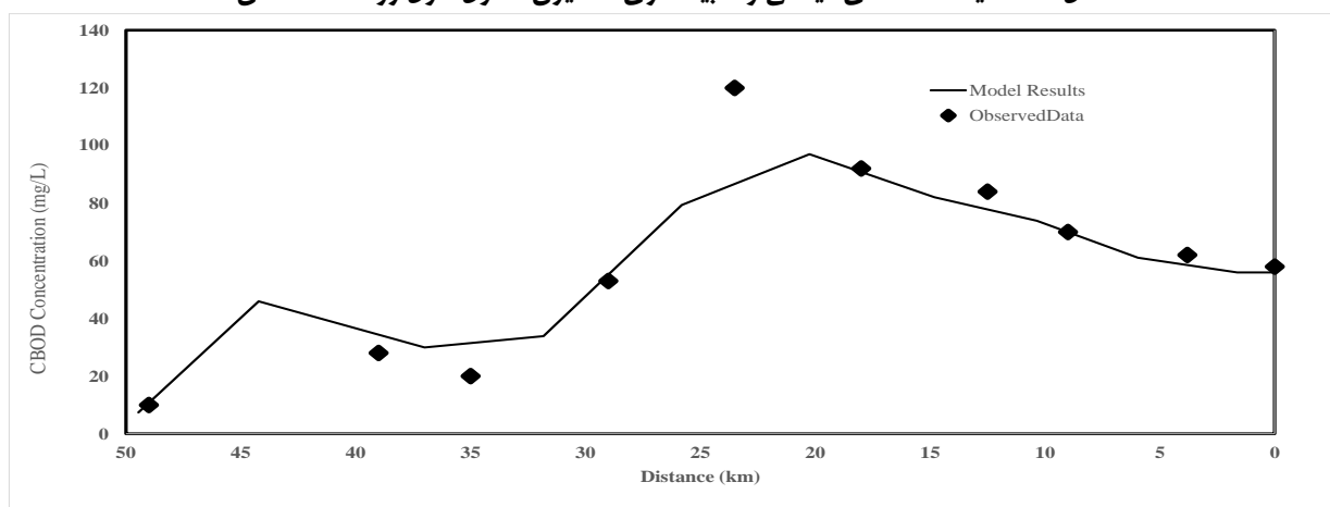
Fig. 4- Comparison simulation results and observed data of CBOD along Geshlagh River شکل ۴- مقایسه CBOD شبیه‌سازی شده و داده‌های میدانی طول رودخانه قشلاق
