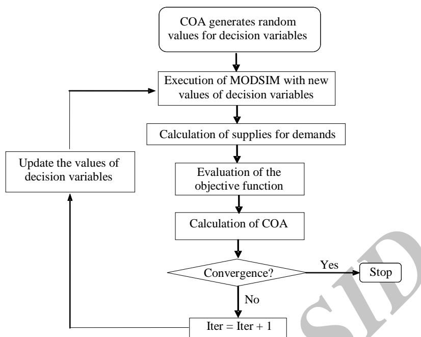
Fig. 1- Flowchart of the COA-MODSIM coupled model شکل ۱- روندنمای عملکرد مدل COA-MODSIM
