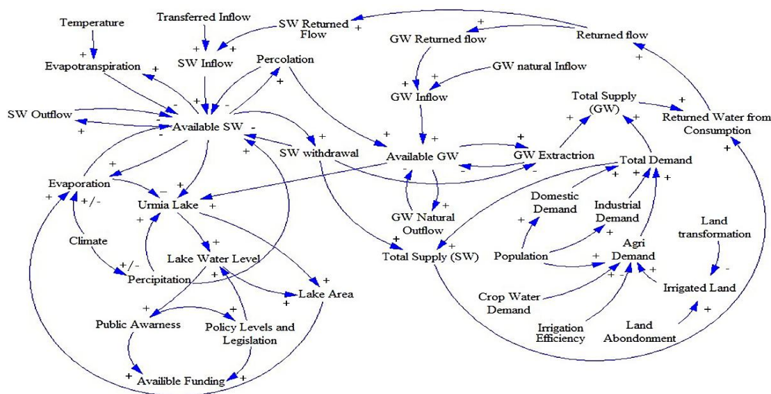
Fig. 2- Casual loop diagram for Urmia Lake شکل ۲- نمودار علت و معلولی دریاچه ارومیه
