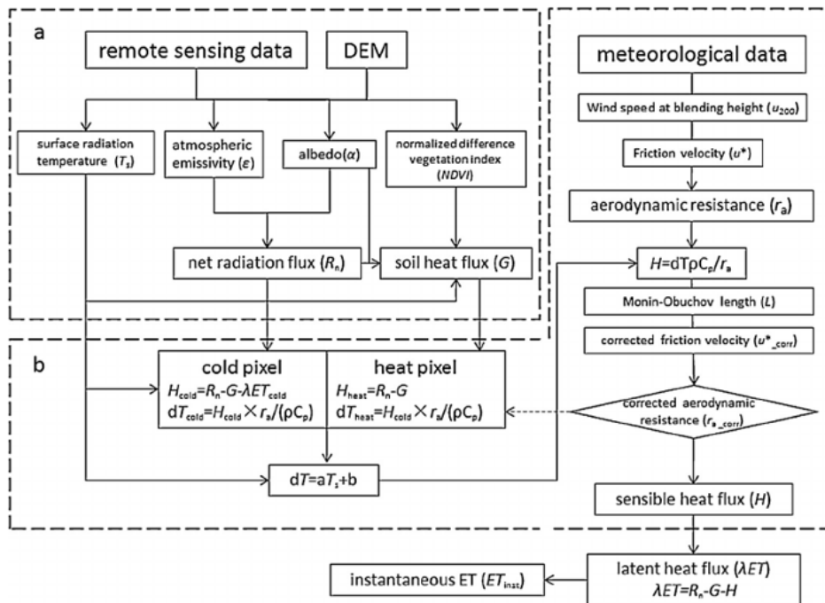
Fig. 2- The flowchart of SEBAL method for calculating evapotranspiration (Bastiaanssen et al., 1999) شکل ۲- فلوجارت روش سبال برای محاسبه تبخیر- تعرق
