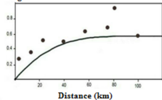
Fig. 2- Fitted exponential variogram on the data شکل ۲- نیم تغییرنا نمای برازش داده شده بر روی داده‌ها
