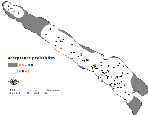
Fig. 3- Spatial distribution of the acceptance probability values and location of existing wells شکل ۳- توزیع مکانی مقادیر احتمال پذیرش و موقعیت چاه‌های موجود
