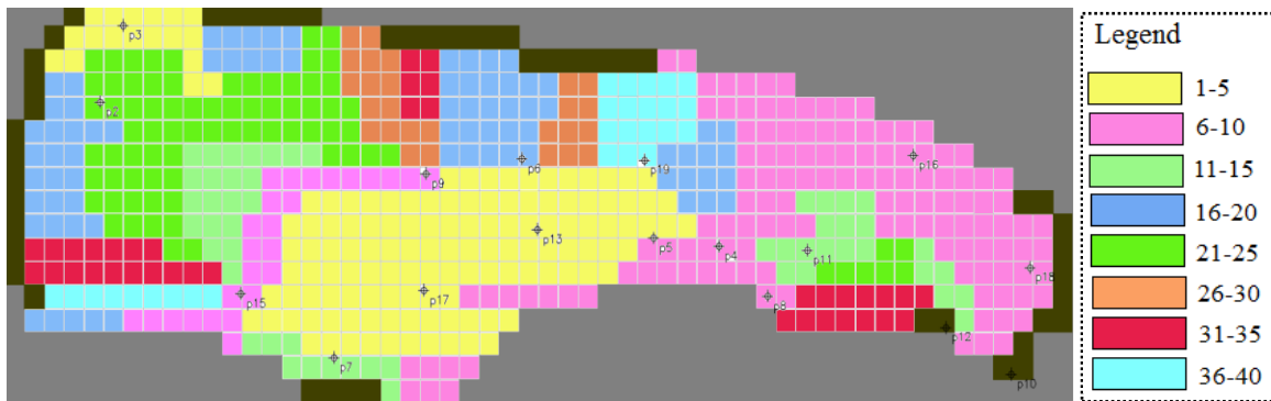
Fig. 4- Zoning map of hydraulic conductivity in PMWIN model شکل ۴- نقشه پهنه‌بندی پارامتر هدایت هیدرولیکی در مدل PMWIN
