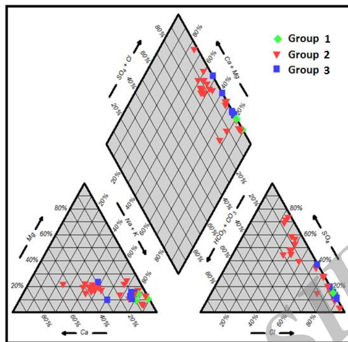
Fig. 4- Piper diagram of the Bostan plain water samples شکل ۴- نمودار پایپر نمونه‌های تجزیه و تحلیل شده منابع آب دشت بستان
