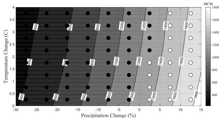
Fig. 4- Lake inflow under climate scenarios شکل ۴ - حجم آب ورودی به دریاچه تحت سناریوهای اقلیمی
