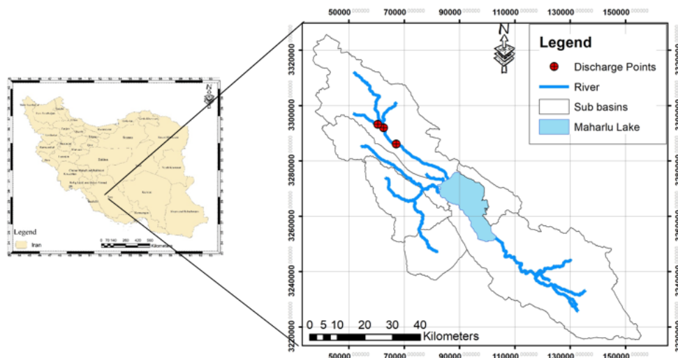
Fig. 1- Location of the case study area, riverine network and hydrometric stations in Maharlu Basin شکل ۱- موقعیت مکانی حوضه دریاچه مهارلو، ایستگاه‌های آبسنجی و رودخانه‌ها در حوضه دریاچه مهارلو
