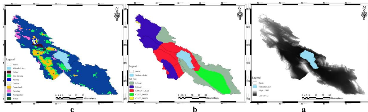
Fig. 2- Map of DEM (a), Soil (b) and Land Use (c) in Maharlu Basin شکل ۲- نقشه DEM (a)، خاک (b) و کاربری اراضی (c) در حوضه مهارلو
