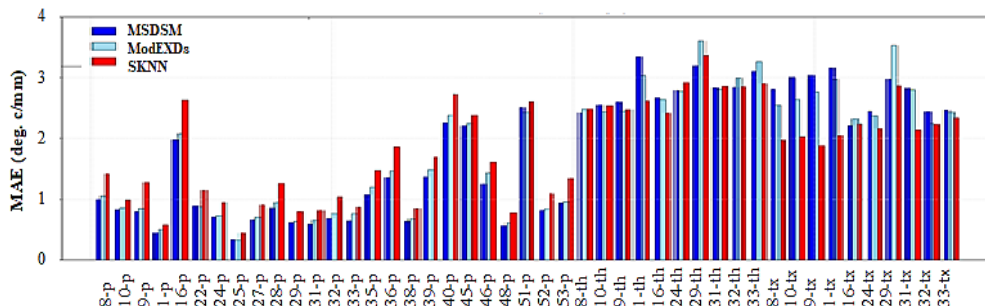
Fig. 3- Mean absolute error diagram of observed and simulated values in observation station (198-2011) شکل ۳- نمودار میان MAE خطای مطلق مقادیر مشاهداتی و شبیه‌سازی شده ایستگاه‌های مشاهداتی طی دوره اعتبارسنجی (۱۹۸۲-۲۰۱۱)
