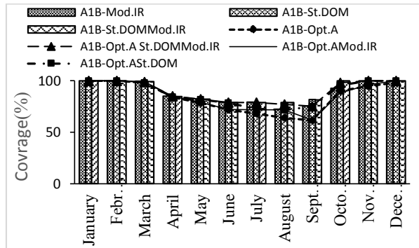
Fig. 14- Coverage of agricultural water needs شکل ۱۴- درصد تأمین نیاز آب کشاورزی
