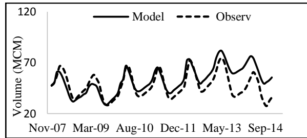
Fig. 11- The monthly observed and simulated storage in Sattarkhan Dam (MCM) شکل ۱۱- میانگین ماهانه مقادیر مشاهده‌ای و شبیه‌سازی شده حجم مخزن سد ستارخان بر حسب (MCM)
