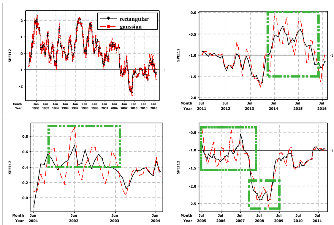
Fig. 8- Time series graph of SPEI12 at Murchekhort station شکل ۸- نمودار سری زمانی شاخص SPEI دوازده ماهه ایستگاه مورچه خورت
