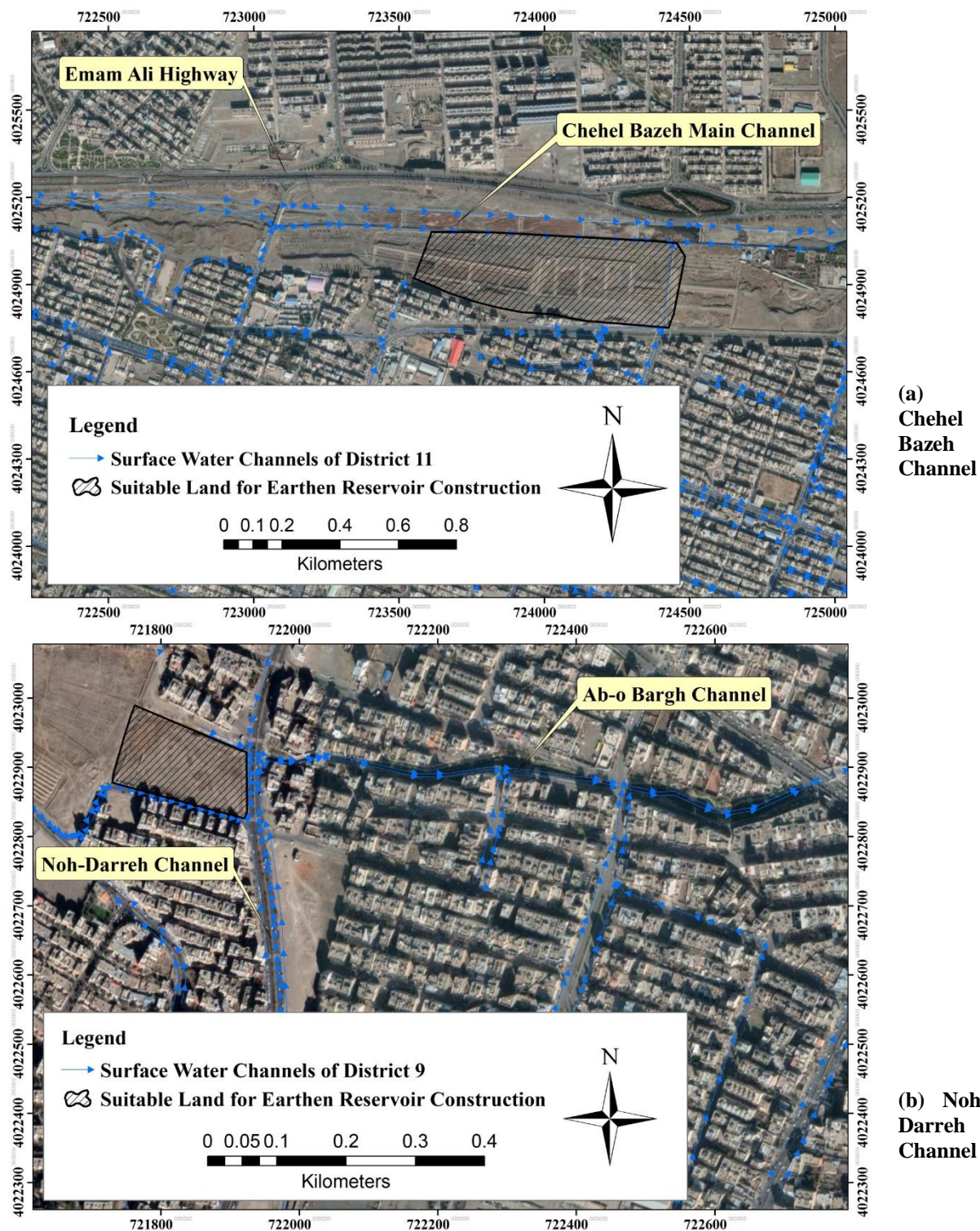
Fig. 6- The location of the proposed earthen water reservoirs with a volume of 30,000 \text{ m}^3 شکل ۶- موقعیت مخازن خاکی پیشنهادی با حجم 30,000 متر مکعب
