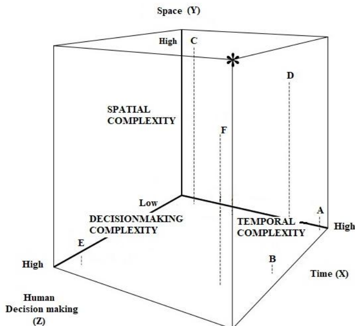
Fig. 2- Three-dimensional framework for reviewing and assessing models of land-use change شکل ۲- چارچوب سه بعدی برای بررسی و ارزیابی مدل‌های تغییر کاربری زمین (Agarwal et al., 2002)
