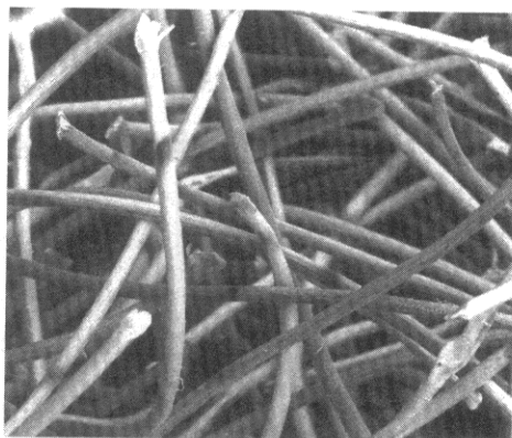
شکل ۳- تصویر SEM الیاف PAN تجاری.
