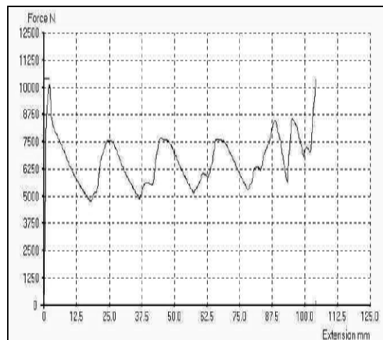
شکل ۶- نمودار تست سلول چهارگوش برنجی با عرض خارجی ۲۰mm، ضخامت ۱ mm و ارتفاع ۱۵۰ mm.
