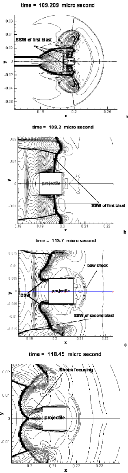
شکل (۷): خطوط هم‌تراز عدد ماخ هنگام گذر پرتابه از موج ضربه‌ای ثانویه انفجاری اول.
