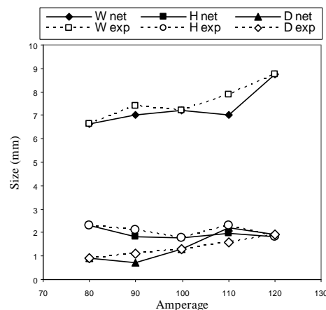
شکل (۵): نمودار مقایسه اثر تغییرات آمپر بر هندسه جوش و در سرعت ۱۲۵ mm/min (خطوط توپر نتایج شبکه و خطوط نقطه‌چین نتایج آزمایش می‌باشند).
