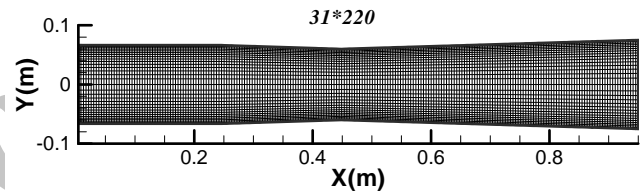
Nozzle C---P0=25 KPa---T0=358.6 K
