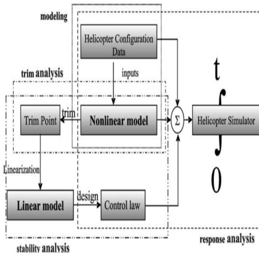
شکل (۲): بلوک دیاگرام کنترل برای شبیه‌سازی [۱].
