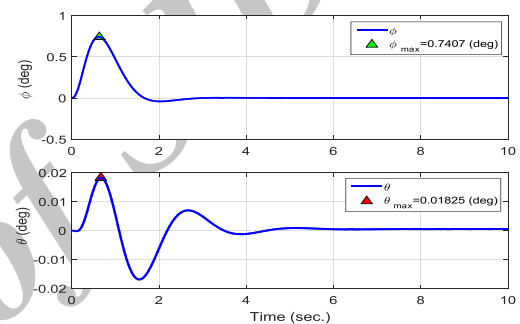
شکل (۱۸): پاسخ زوایای اویلر به ورودی پله اعمالی در
