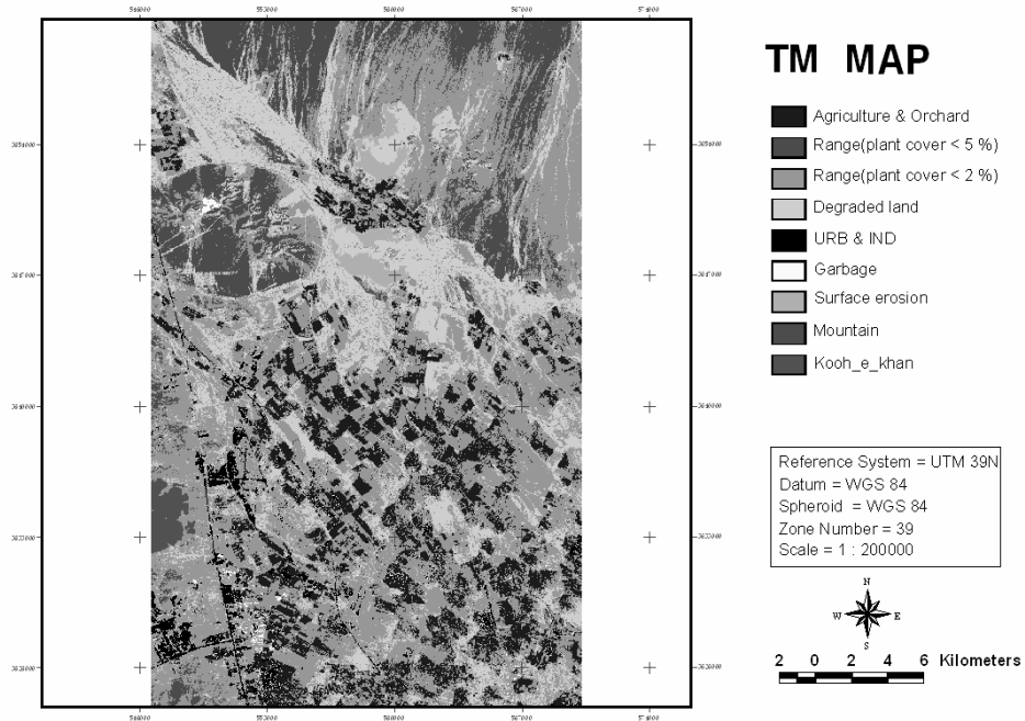
شکل ۳- تصویر ماهواره ETM + طبقه بندی شده
