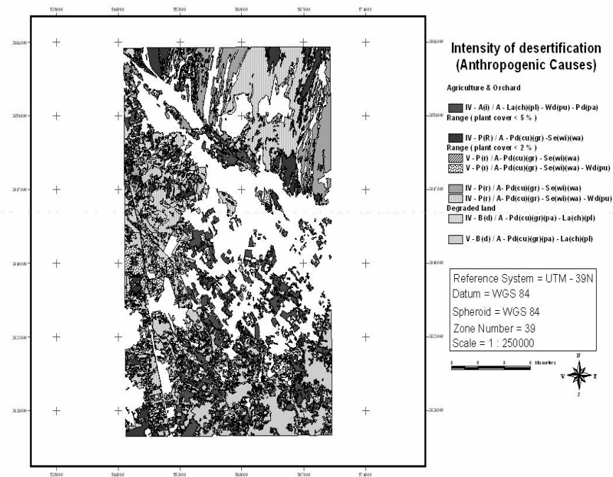
شکل ۶- نقشه شدت بیابان زایی با عوامل انسانی
