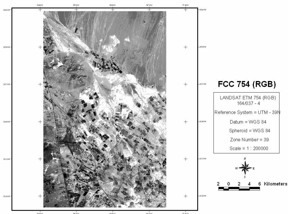
شکل ۱- تصویر ماهواره ETM^+ با ترکیب باندهای ۷۵۴
