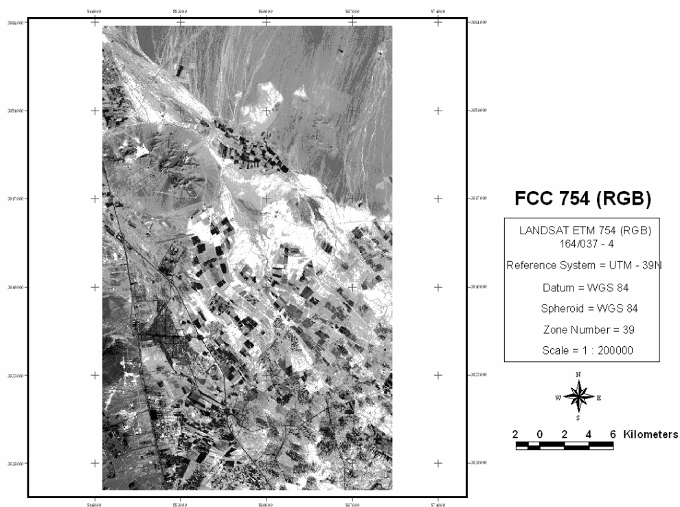
شکل ۲- تصویر ماهواره TM طبقه بندی شده
