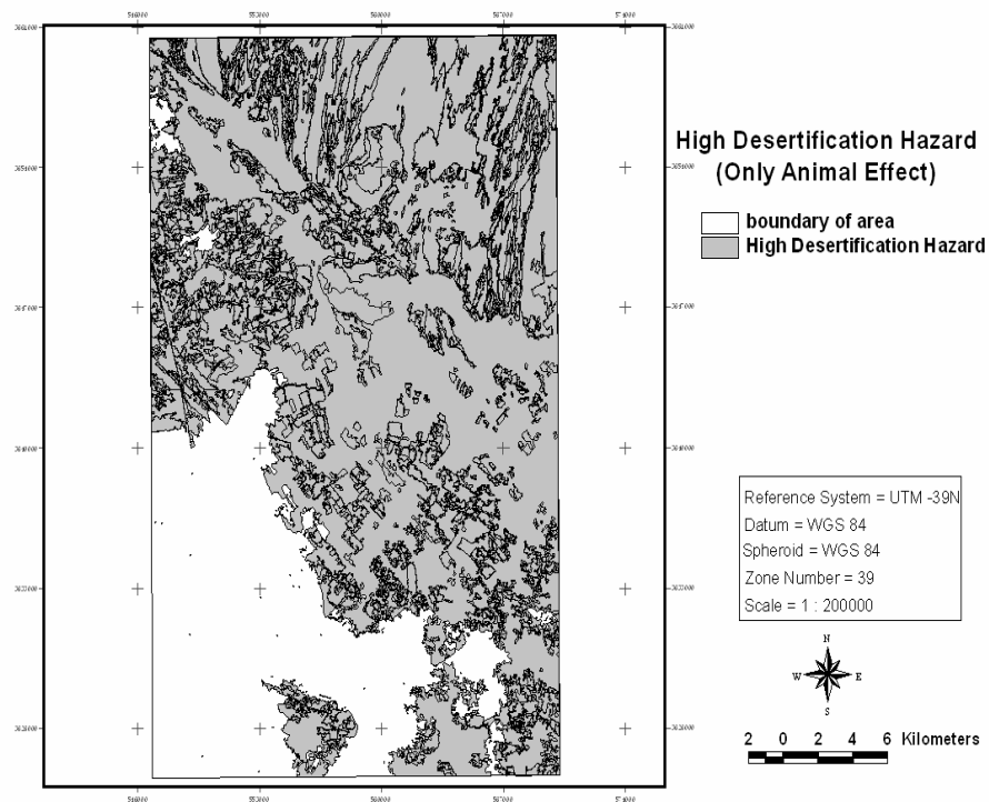
شکل ۸- نقشه خطر بیابان زایی باتاثیر جمعیت دام
