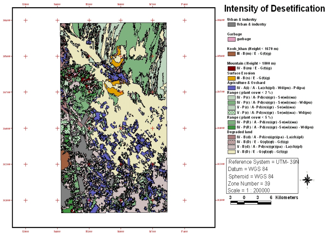
شکل ۴- نقشه شدت بیابان زایی
