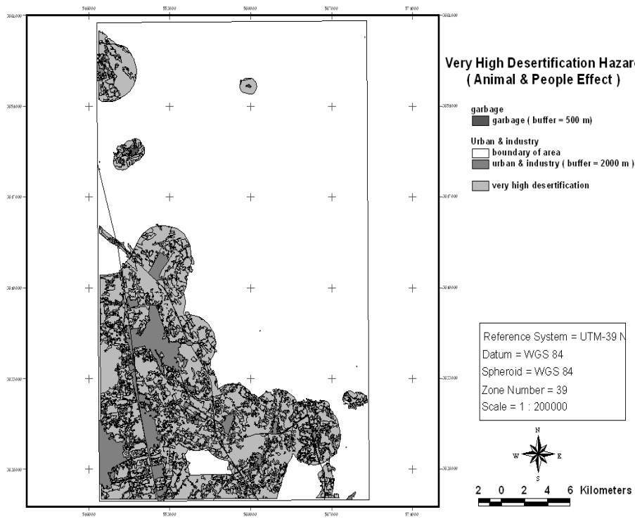
شکل ۷- نقشه خطر بیابان زایی باتاثیر جمعیت انسانی و دام
