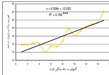
نمودار ۷- روند تغییرات میانگین لغزان ضریب رواناب پاییزه آبخیز رودخانه کردان در هم‌دوره ۳۰ ساله ۷۴-۷۵ / ۴۶-۴۵.۱۳۴۵
