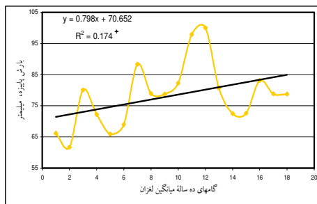
نمودار ۴- روند تغییرات میانگین لغزان بارش پاییزه آبخیز رودخانه کردان در همدوره ۳۰ ساله ۷۵-۷۴ / ۴۶-۴۵.
