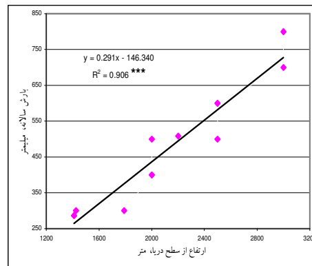
نمودار ۱- همبستگی بارش سالانه و ارتفاع در آبخیز رودخانه کردان.
