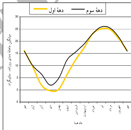
نمودار ۹- تغییرات میانگین ماهانه دمای روزانه هوای ایستگاه سینوپتیک کرج در دهه های اول و سوم هم‌دوره ۳۰ ساله ۷۴-۷۵ / ۴۶-۴۵.۱۳۴۵ (به تقویم خورشیدی).
