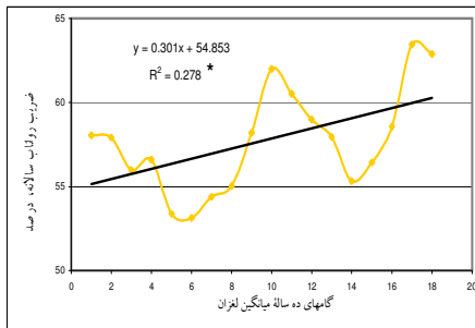
نمودار ۸- روند تغییرات میانگین لغزان ضریب رواناب سالانه آبخیز رودخانه کردان در هم‌دوره ۳۰ ساله ۷۴-۷۵ / ۴۶-۴۵.۱۳۴۵
