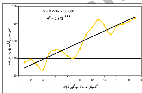
نمودار ۶- روند تغییرات میانگین لغزان ضریب رواناب بهاره آبخیز رودخانه کردان در همدوره ۳۰ ساله ۷۵-۷۴ / ۴۶-۴۵.
