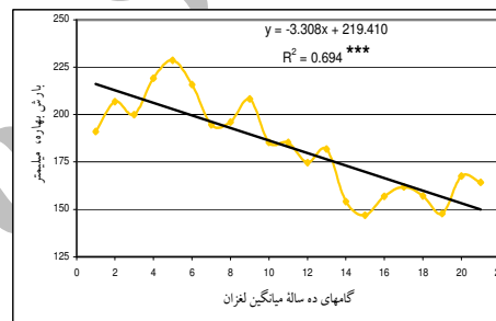
نمودار ۳- روند تغییرات میانگین لغزان بارش بهاره آبخیز رودخانه کردان در همدوره ۳۰ ساله ۷۵-۷۴ / ۴۶-۴۵.
