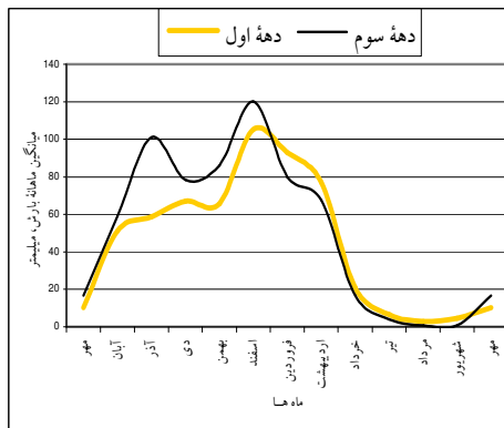
نمودار ۲- تغییرات پراکنش ماهانه بارش آبخیز رودخانه کردان در دهه‌های اول و سوم از همدوره ۳۰ ساله ۷۵-۷۴ / ۴۶-۴۵ (دقت برررسیهای منبع آب).
