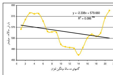
نمودار ۵- روند تغییرات میانگین لغزان بارش سالانه آبخیز رودخانه کردان در همدوره ۳۰ ساله ۷۵-۷۴ / ۴۶-۴۵.
