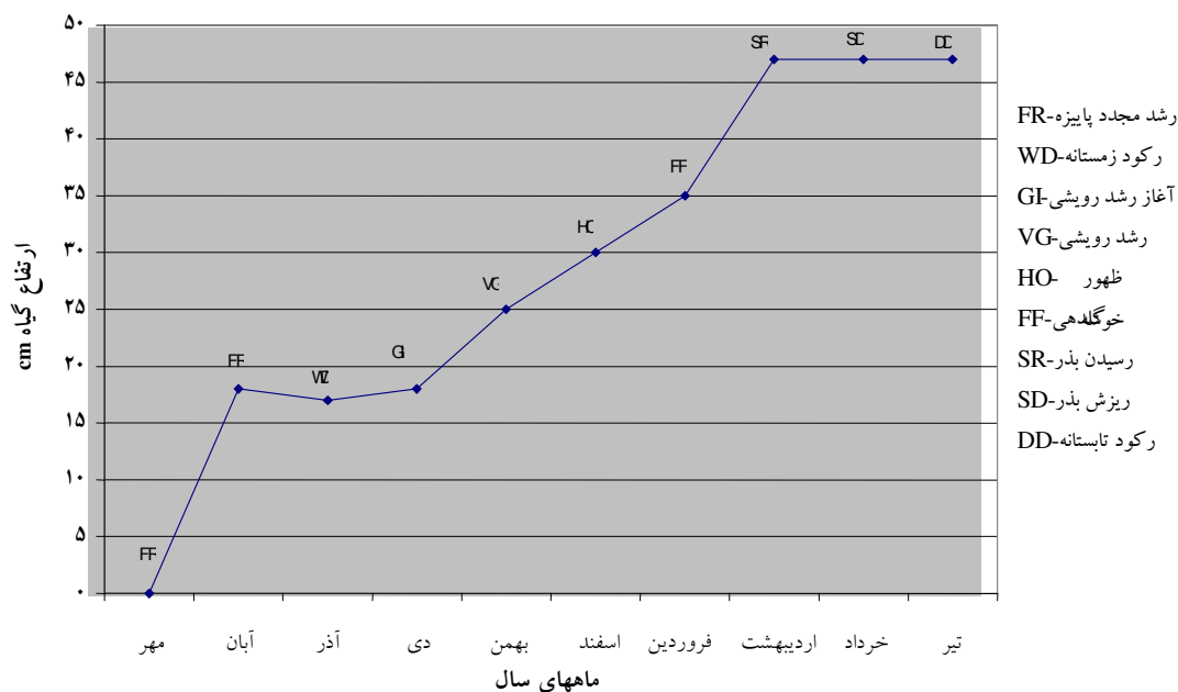
شکل ۲- نمودار مراحل حیاتی گونه مرتعی Cenchrus ciliaris
