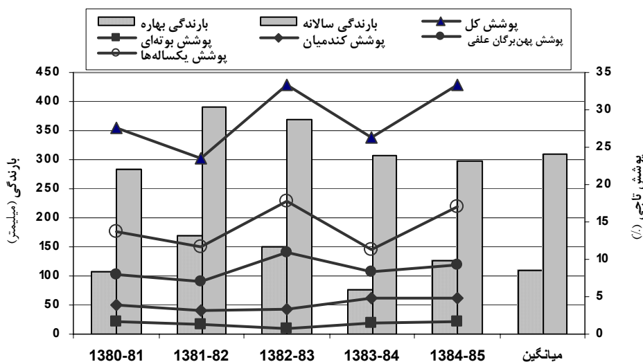
شکل ۲- تغییرات بارندگی و پوشش تاج کل و فرمهای رویشی در قرق ارکوتین در سالهای ۸۵-۱۳۸۱
