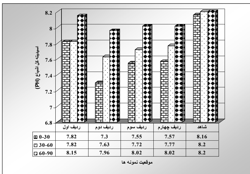
شکل ۴- مقایسه تغییرات pH (اسیدیته کل اشباع) ردیف‌های نمونه‌گیری با شاهد در اعماق ۰-۳۰، ۳۰-۶۰، ۶۰-۹۰ سانتی متری خاک
