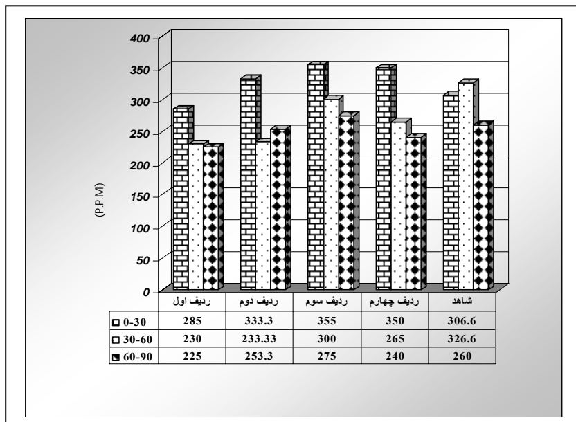
شکل ۱۰- مقایسه تغییرات پتاسیم قابل جذب رذیف‌های نمونه‌گیری با شاهد در اعماق ۰-۳۰، ۳۰-۶۰ و ۶۰-۹۰ سانتی متری خاک
