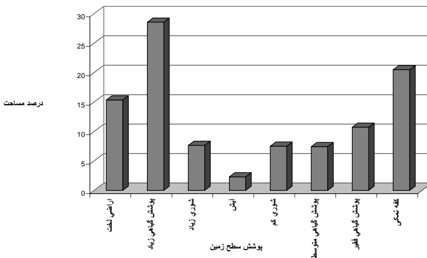
شکل ۲- مساحت پوشش‌های سطح زمین (مستخرج از نقشه‌های پوشش سطح زمین)
