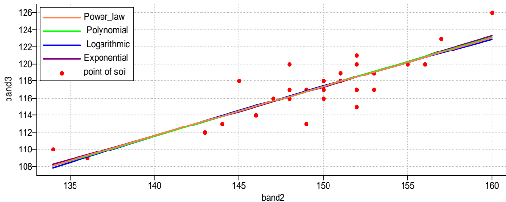
شکل ۳- نمودار معادله خط خاک با روشهای مختلف برازش
