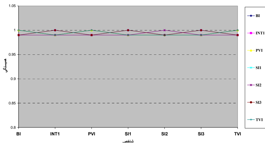
شکل ۱۳ - همبستگی شاخص‌های با قابلیت بارزسازی شوری
