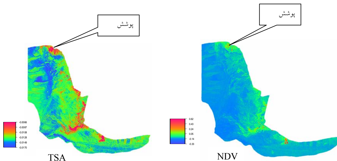
شکل ۴- شاخص NDVI بدون قابلیت بارزسازی پوشش گیاهی و شاخص TSAVI دارای قابلیت بارزسازی پوشش گیاهی
