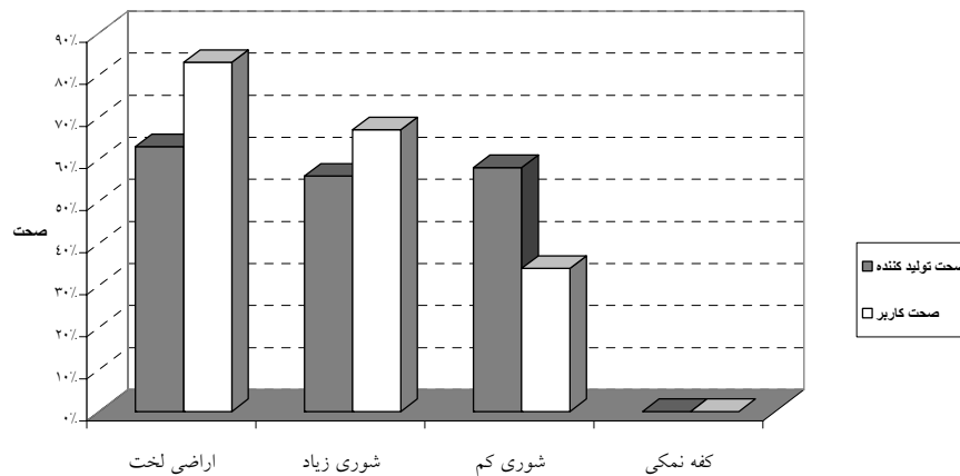
شکل ۱۱- نمودار مقایسه صحت کاربر و تولیدکننده در شاخص‌های بدون قابلیت بارزسازی شوری
