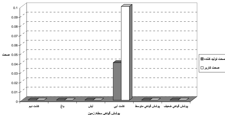
شکل ۶- مقایسه صحت کاربر و تولیدکننده در شاخص‌های بدون قابلیت بارزسازی پوشش گیاهی
