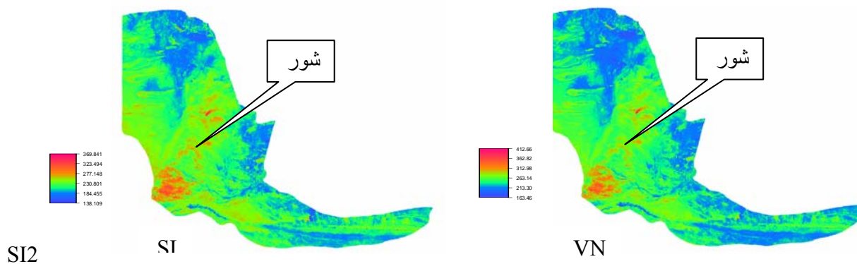
شکل ۹ - شاخص VNIR بدون قابلیت بارزسازی و شاخص SI2 با قابلیت بارزسازی سطح شور
