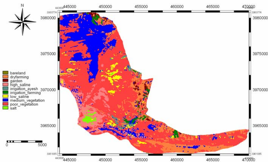
شکل ۷- نقشه پوشش سطح زمین با شاخص‌های توانایی بارزسازی پوشش گیاهی
