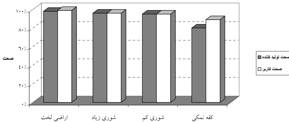
شکل ۱۰- نمودار مقایسه صحت کاربر و تولیدکننده در شاخص‌های با قابلیت بارزسازی شوری
