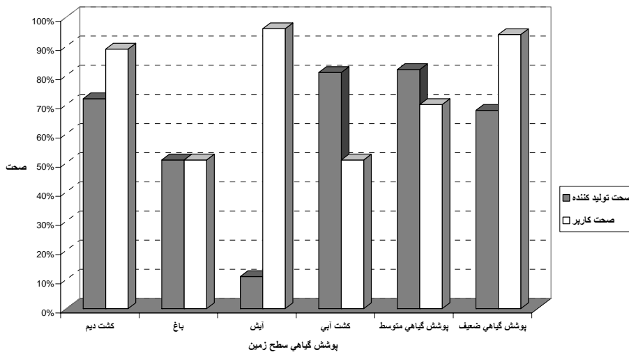
شکل ۵- مقایسه صحت کاربر و تولیدکننده در شاخص‌های با قابلیت بارزسازی پوشش گیاهی
