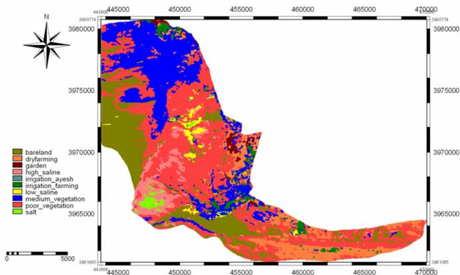
شکل ۱۲ - نقشه پوشش سطح زمین با شاخص‌های توانایی بارزسازی شورزار
