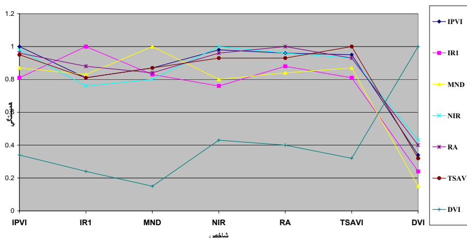
شکل ۸- همبستگی شاخص‌های با قابلیت بارزسازی پوشش گیاهی شاخص‌های شوری
