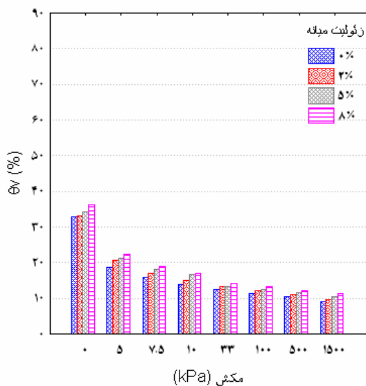
شکل ۲- تغییرات درصد رطوبت حجمی در مکش‌های ۰ تا ۱۵۰۰ کیلو پاسکال در خاک شنی در اثر کاربرد زئولیت کلینوپتیلولیت میانه و سوپرجاذب A200.
