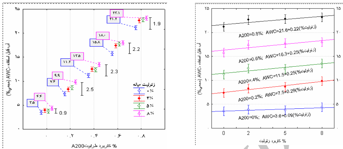
شکل ۴- اثر متقابل کاربرد زئولیت میانه (سمت راست) و سوپر جاذب طراوت A_{200} (سمت چپ) بر آب قابل استفاده در خاک شنی (در نمودار سمت راست رابطه‌ی آب قابل استفاده با درصد کاربرد زئولیت در پنج سطح کاربرد پلیمر دیده می‌شود. در نمودار سمت چپ مقادیر آب قابل استفاده در عدم و کاربرد ۸ درصد زئولیت در پنج سطح کاربرد پلیمر و افزایش آب قابل استفاده در اثر افزودن ۸ درصد زئولیت با ارقام لاتین نشان داده شده است).
