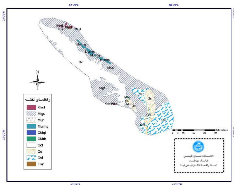
شکل ۴- نقشه زمین شناسی
