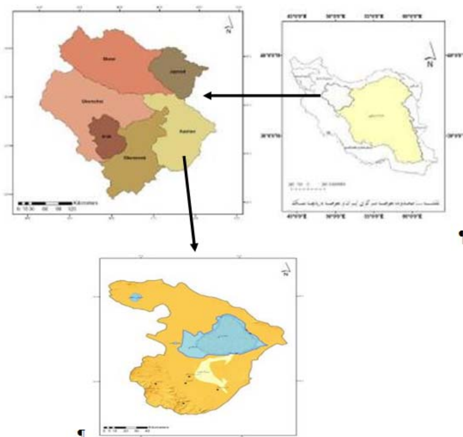
شکل ۱- موقعیت دریاچه نمک و حاشیه مرطوب آن
