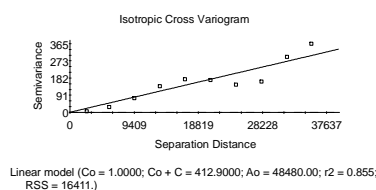
شکل ۱۰- واریوگرام متقابل پوشش تاجی
