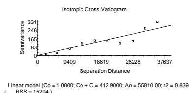
شکل ۹- واریوگرام متقابل تراکم
