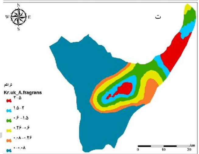
شکل ۶- نقشه‌های تهیه شده بر اساس روش‌های آمار مکانی پارامتر تراکم (پایه در مترمربع) در منطقه مورد مطالعه: الف) روش Inverse Distance Weighting (ب) روش Kr. Simple (پ) روش Kr. Ordinary (ت) روش Kr. Universal (ث) روش Kr. Disjunctive
