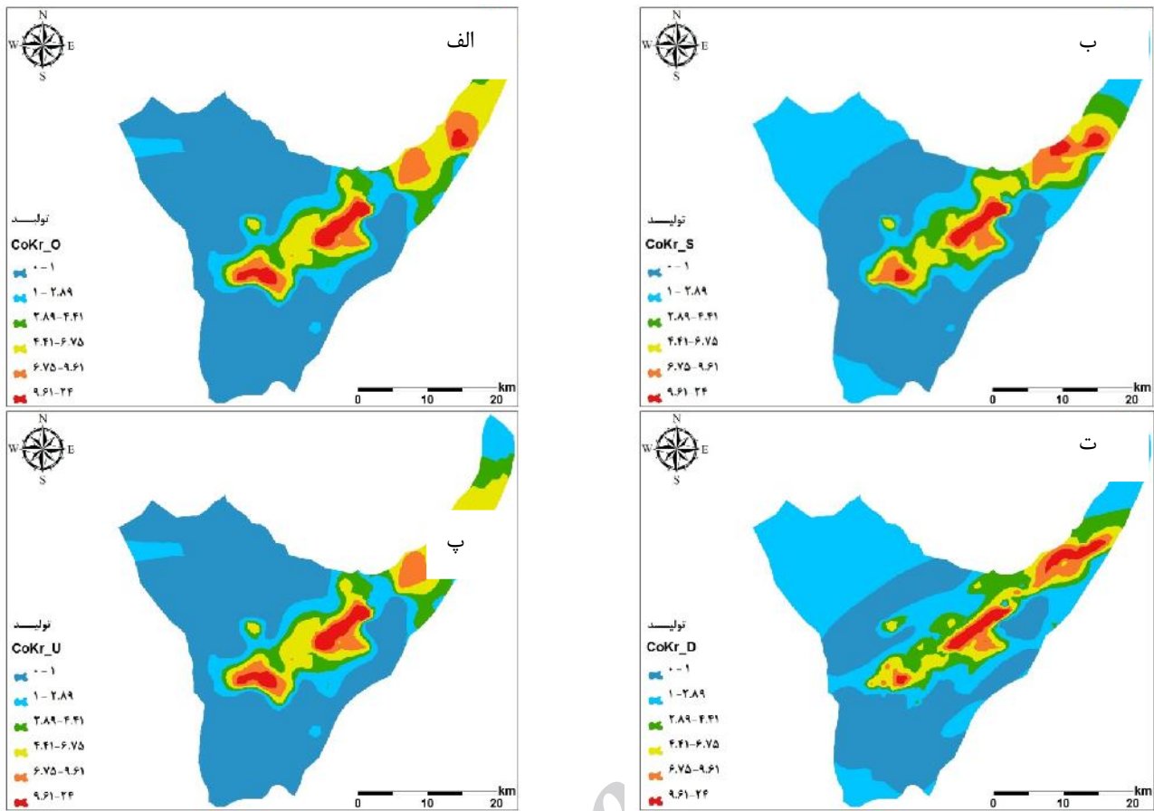
شکل ۱۴- نقشه‌های تهیه شده بر اساس روش‌های آمار مکانی پارامتر تولید (گرم در مترمربع) در منطقه مورد مطالعه: الف) روش CoKr. Ordinary (ب. CoKr. Disjunctive، پ) روش CoKr.Simple، ت) روش CoKr.Universal.
