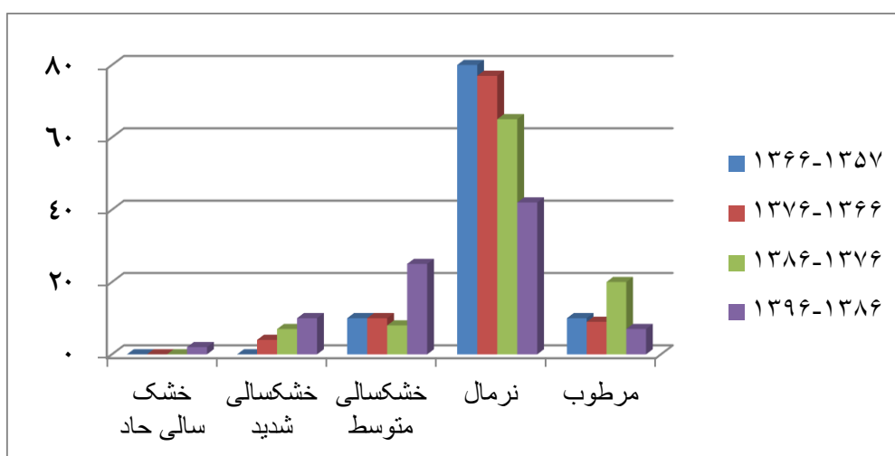
شکل ۳- مساحت انواع خشکسالی در حوزه آبخیز حبله‌رود بر اساس نقشه شاخص spi
