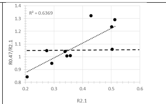
شکل ۴- نسبت باند قرمز و آبی به مادون قرمز میانی سنجنده OLI
