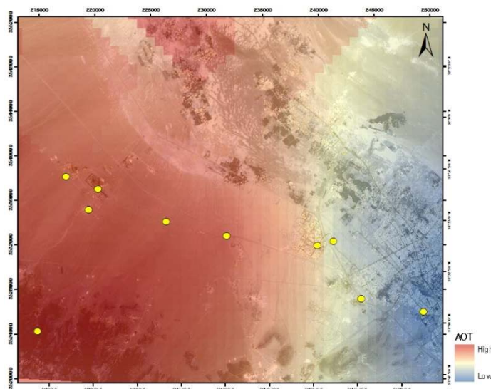
شکل ۶- ضخامت نوری محاسباتی ریزگرد با طول موج ۰/۶۵ میکرومتر (AOT 0.65 \mu m)
