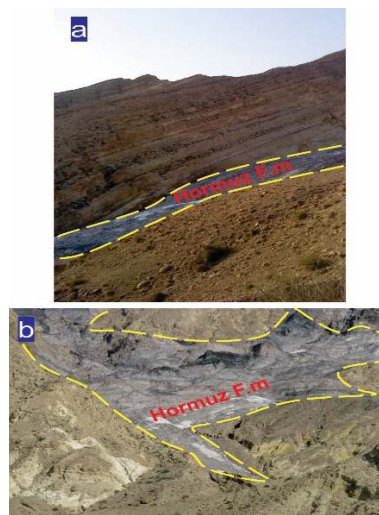
شکل ۳- a: نمکشار طویل جریان یافته در گودال‌های گسلی (دید به سمت شمال غرب)، b: نمکشار جاری شده بر روی سنگ‌های درونگیر و سراسیبه‌ها (دید به سمت شمال)
