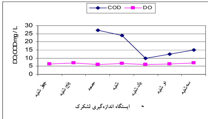
شکل ۴- تغییرات متوسط روزانه COD و DO
