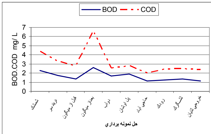
شکل ۱۴- تغییرات COD و BOD در ایستگاه‌های آبفا ۸۱- ۱۳۷۶
