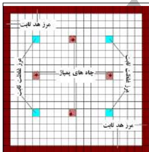
شکل ۴- موقعیت و شرایط مرزی آبخوان
