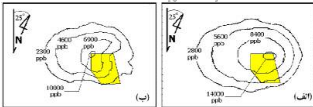
شکل ۸- گسترش نهایی هاله آلودگی (الف: بدون استفاده از عملیات احیاء، ب: با استفاده از عملیات احیاء)
